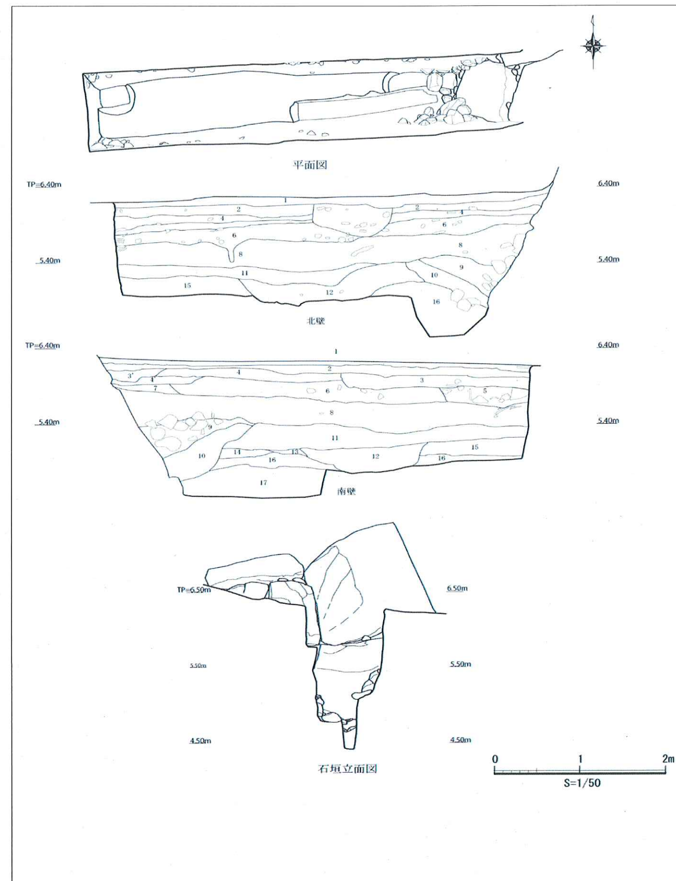
図10 I地点 土層図
