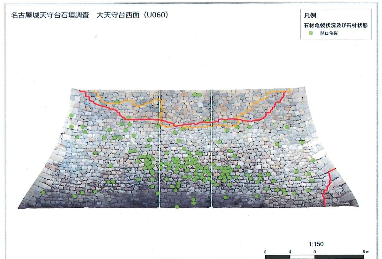
図27 U60石材劣化状況
