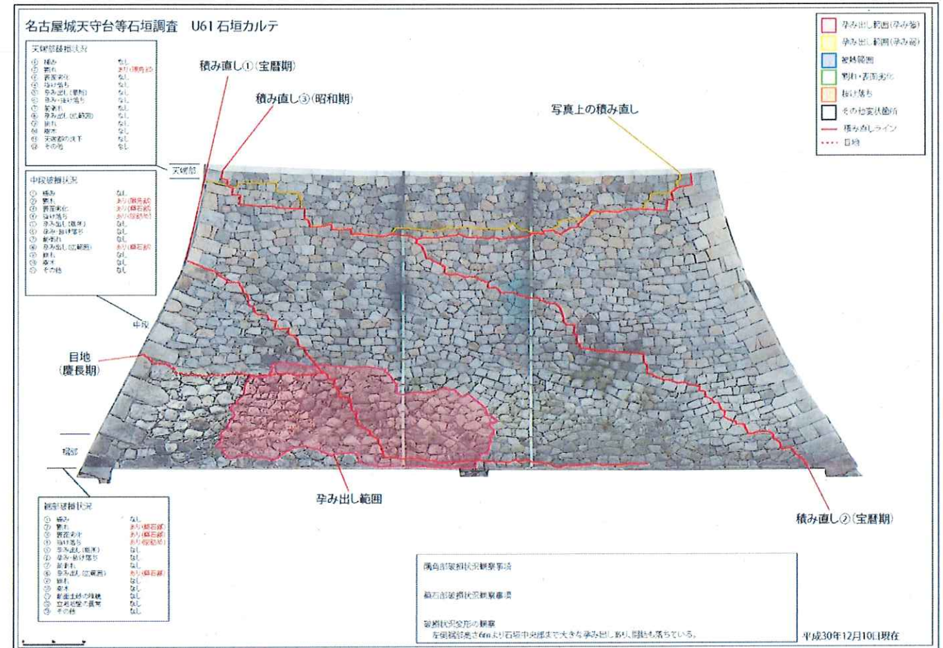
図22 U61石垣カルテ
