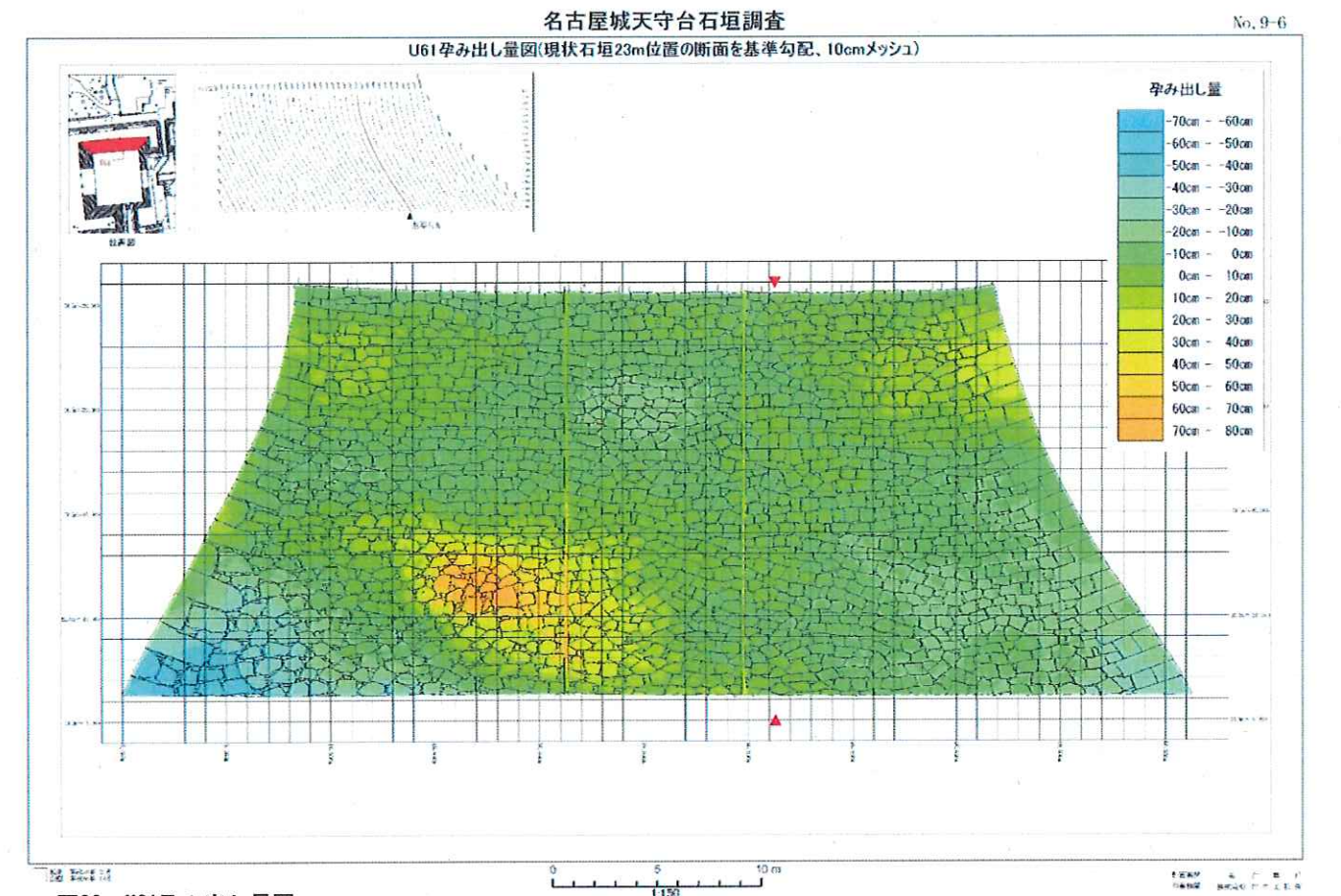
図23 U61孕み出し量図
