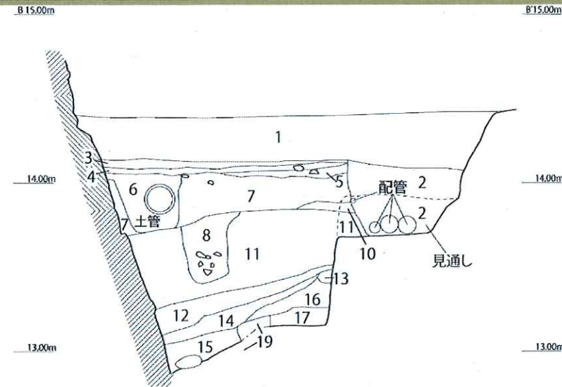
図14 P区東壁セクション
