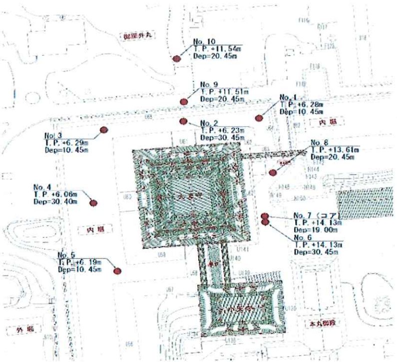
図17 ボーリング調査地点位置図
