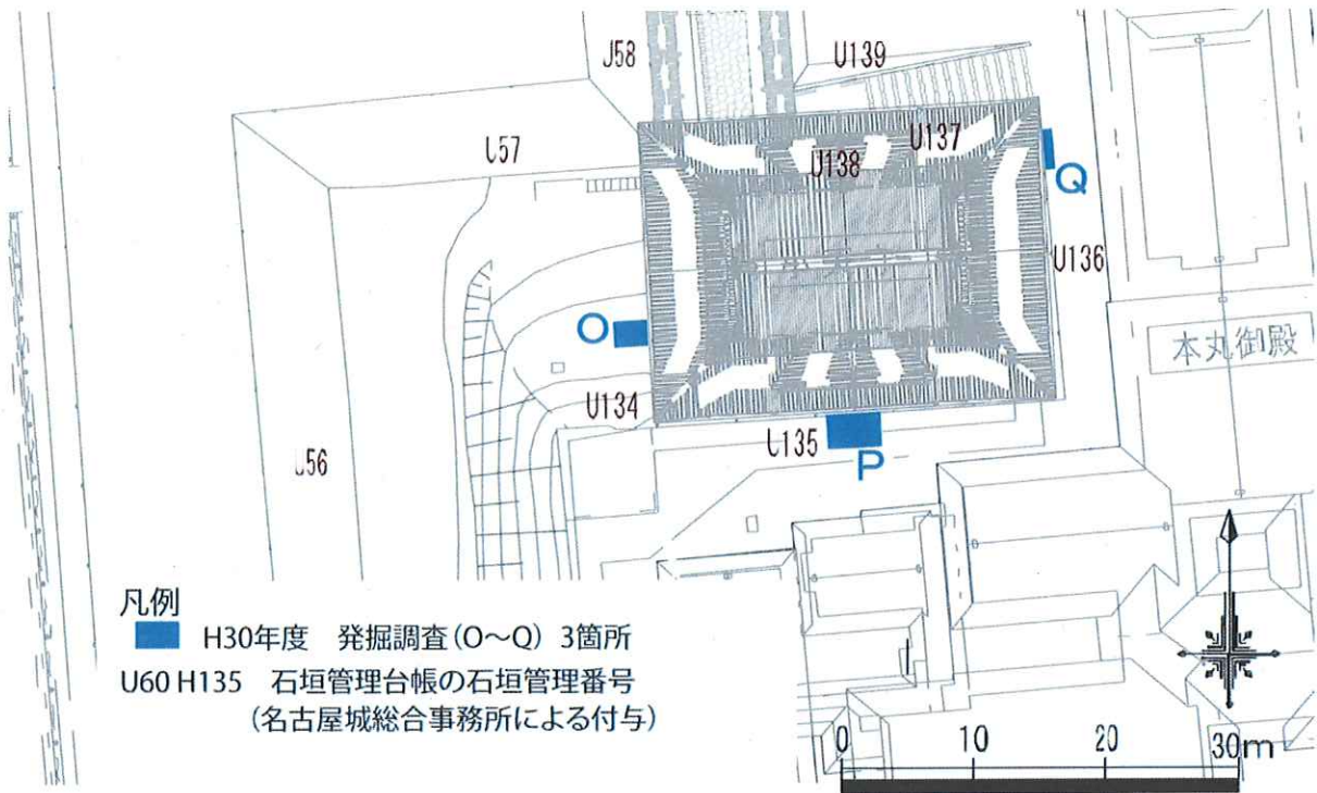
図12 小天守台周辺 調査区位置図
