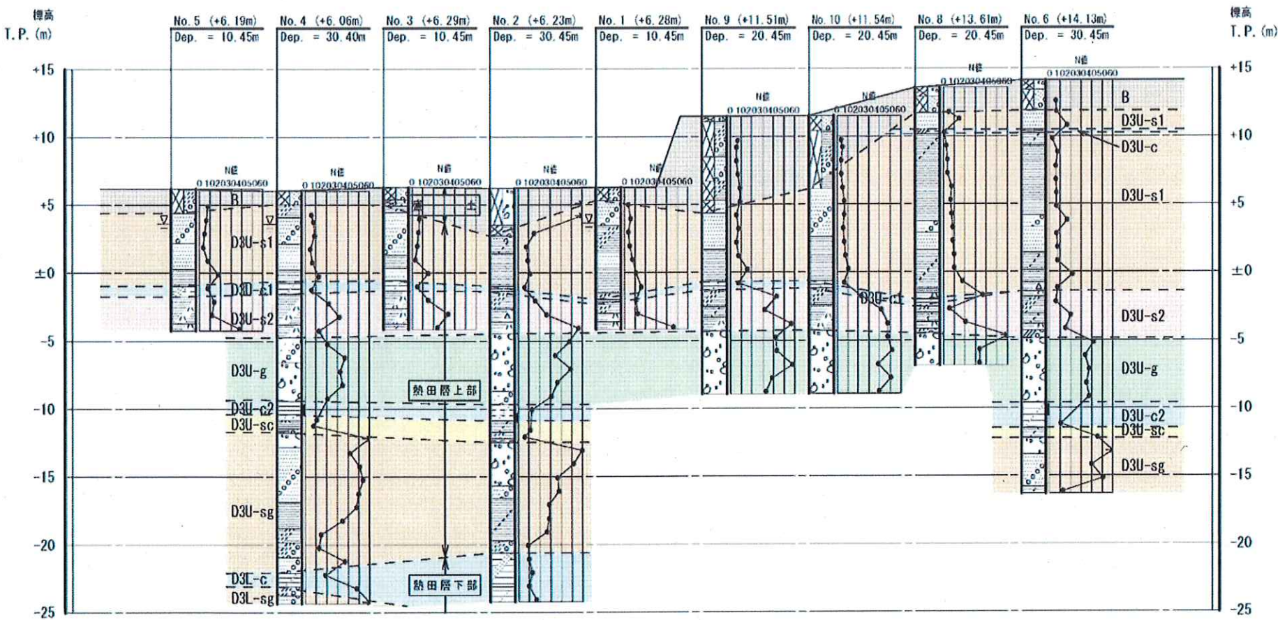
図18 土層（地層区分）想定断面図
