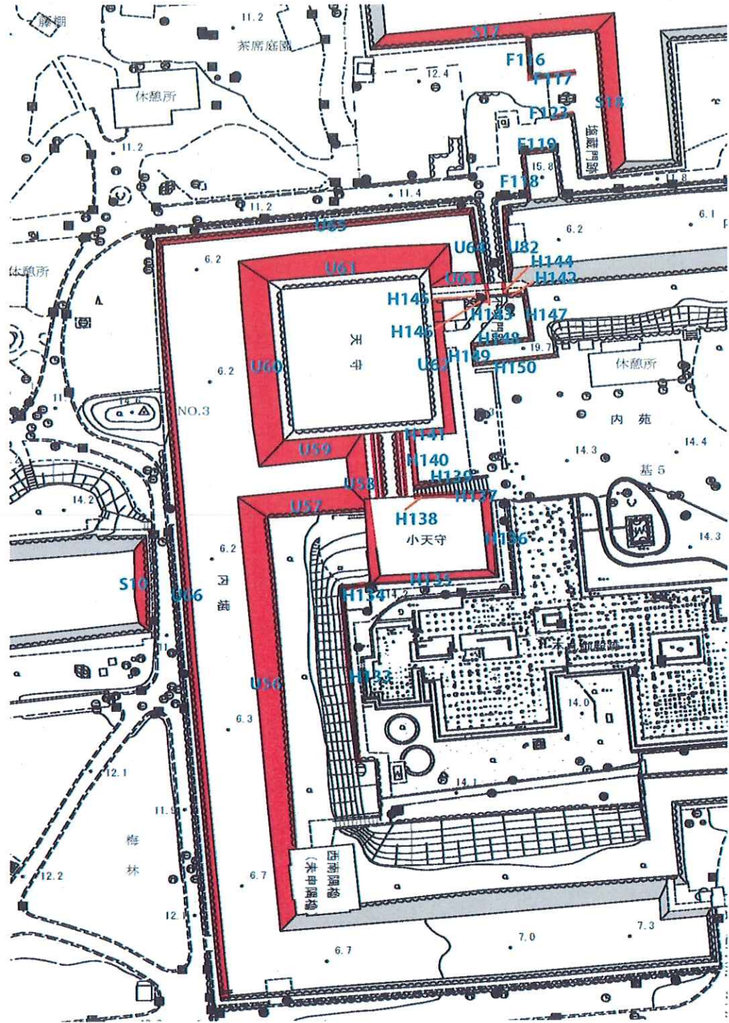
図1 天守台外部石垣管理番号
