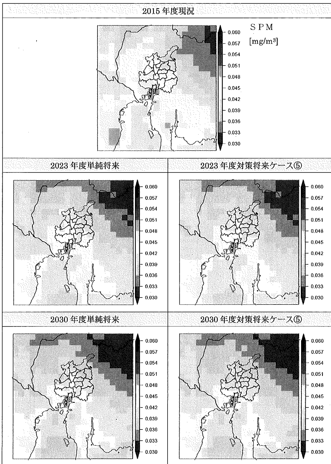
図 1-4 濃度分布図 (SPM : 日平均値の 2% 除外値)
