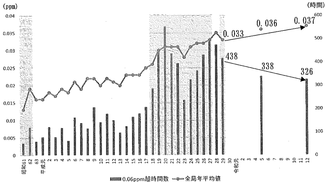
図1 O x の測定結果および将来予測
