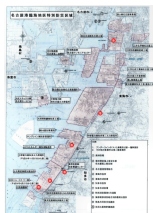
名古屋港地区特別防災区域 泡消火剤貯留施設
