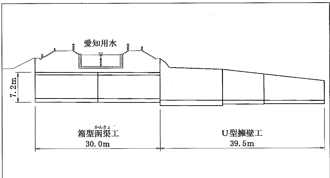
(2) 側面図
