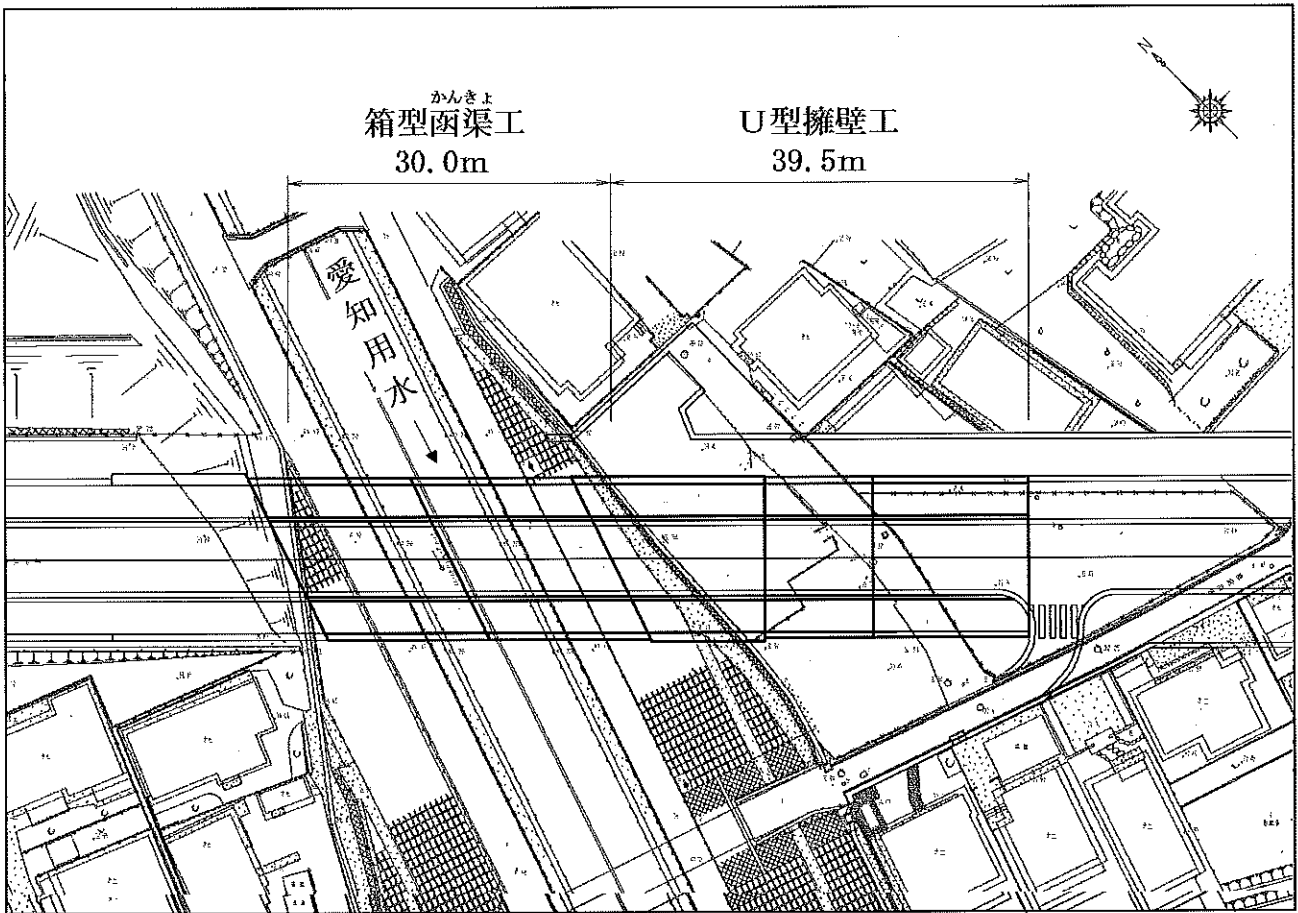
(1) 平面図
